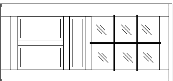
Door 950x2080
